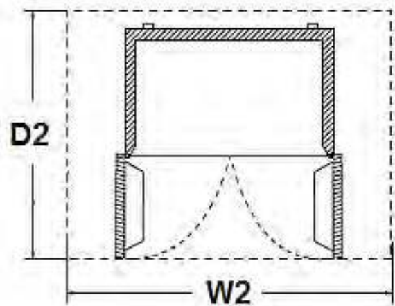
GEÖFFNET
